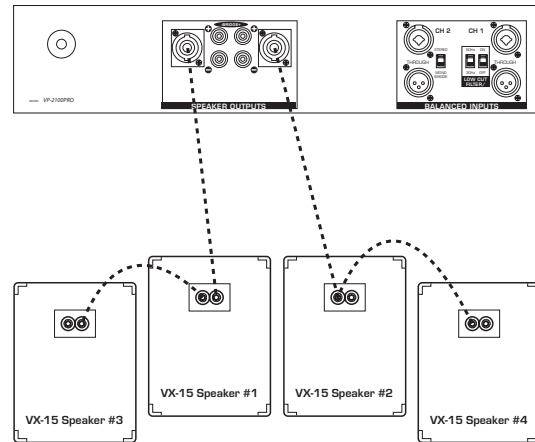
VP-2100 PRO Amplifier
