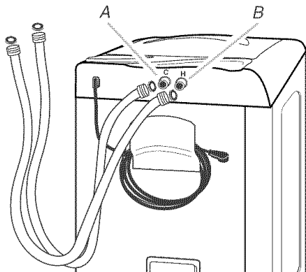
A. Electrovanne d'alimentation - bleue = eau froide B. Electrovanne d'alimentation - rouge = eau chaude
