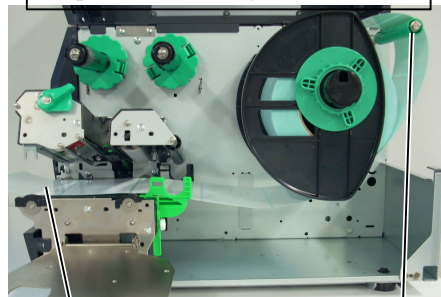
Guide Shaft
