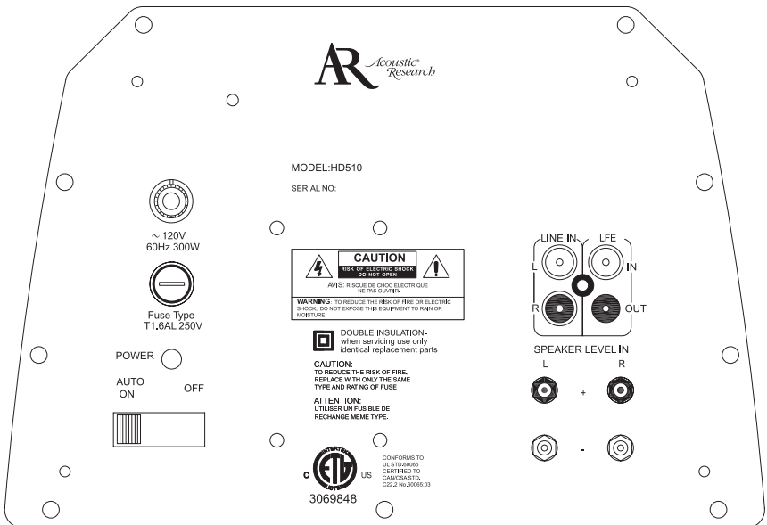
FIGURA 3 - Controles y Conexiones del Altavoz de Subwoofer
