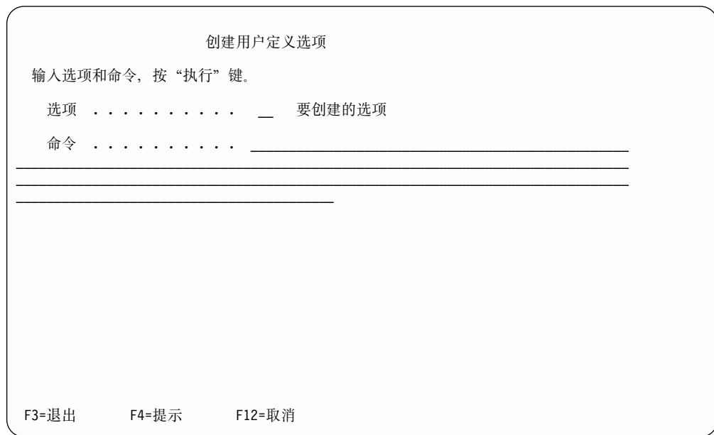
图 87. 创建用户定义选项屏幕
