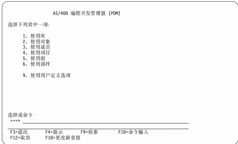
图 63. AS/400 编程开发管理器 (PDM) 主菜单
