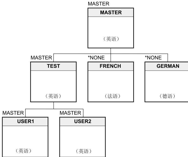
图 88. 用于翻译的项目层次结构
