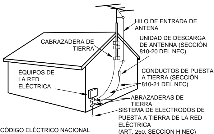
Puesta a tierra de una antena, según el Código Eléctrico Nacional
