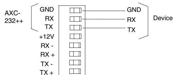
FIG. 2 RS-232 wiring
