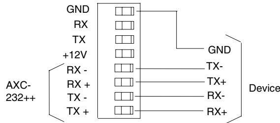
FIG. 3 RS-422 wiring
