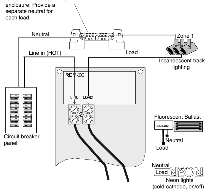
FIG. 3 RDM-ZC wiring configuration
