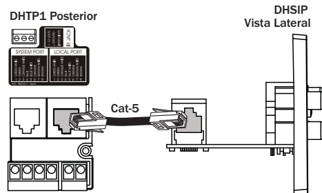
Dibujo 3.6: DHSIP al DHTP1 – Conexiones de atrás
