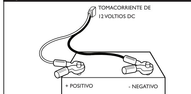
Figura 17 — Conexiones de la Batería
