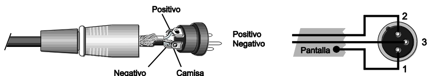
Entrada balanceada
