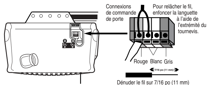
Dénuder le fil sur 7/16 po (11 mm)
