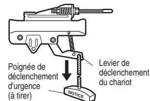
POSITION DE DÉCLANCHEMENT MANUEL
