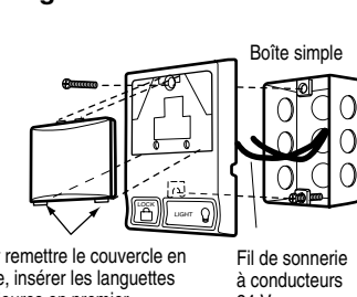
Figure 2 INSTALLATION PRÉCÂBLÉE
