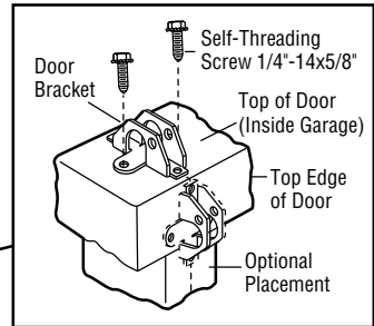
METAL DOOR
