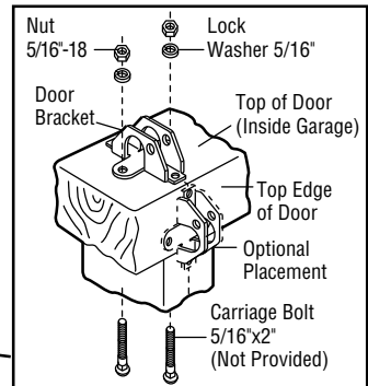
WOOD DOOR
