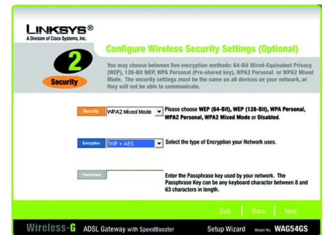
Abbildung 5-29: Setup-Assistent – Fenster Configure Wireless Security Settings (Optional) (Konfigurieren der Wireless-Sicherheitseinstellungen [optional]) – WPA2 Mixed Mode (WPA2 Gemischter Modus)
