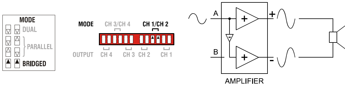
Abbildung 2.4: Betriebsart BRIDGED
