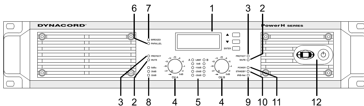
Illustration 2.1 : Face avant du H2500/H5000
