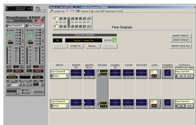
Abbildung 4.2: Bedienpanel und DSP-Flussdiagramm in IRIS-Net™
