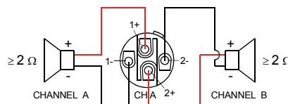
Illustration 2.15 : Connexion de haut-parleur Bi-Amp en mode de fonctionnement NORMAL, uniquement à l'aide du connecteur Speakon A
