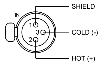
Illustration 4.4: Câblage de la prise AES/EBU-IN
