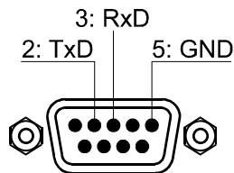
Illustration 4.8: Câblage de l'Interface RS-232
