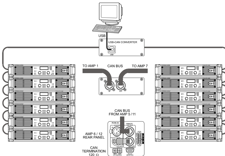
Illustration 4.11: Système avec avec 2 amplis en rack et un UCC-1 au milieu. Bouchons de terminaison sur l'ampli de puissance 6 (première unité du bus) et sur l'ampli de puissance 12 (dernière unité du bus)
