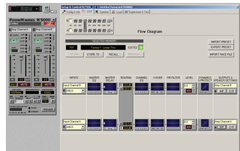
Illustration 4.2: Schéma de principe DSP du module RCM-26
