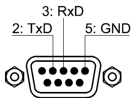
Abbildung 4.8: Belegung der RS-232-Schnittstelle
