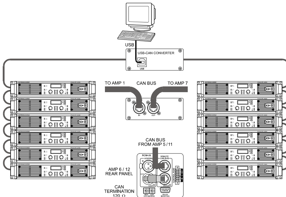
Abbildung 4.11: System mit 2 Racks und einem USB-CAN-Converter. Abschluss-Stecker am Remote-Amplifier 6 (Bus-Anfang) und Remote-Amplifier 12 (Bus-Ende)
