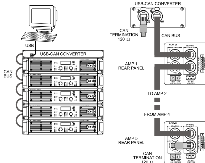
Abbildung 4.10: 5 Remote-Amplifier (mit RCM-26) und ein USB-CAN-Converter am Bus-Anfang. Abschluss-Stecker am USB-CAN-Converter und am RCM-26 des Remote-Amplifier 5
