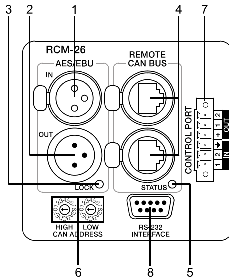
Illustration 4.3: Commandes et connexions RCM-26
