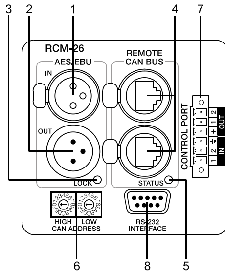
Abbildung 4.3: Bedienelemente und Anschlüsse des RCM-26
