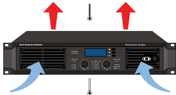
Abbildung 2.6: H2500/H5000 Kühlung
