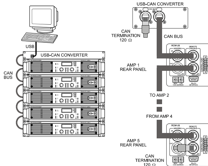
Illustration 4.10: Système avec 5 amplis de puissance et un UCC-1 au début de la chaîne (bus). Bouchons de terminaison sur le UCC-1 (première unité du bus) et sur l'ampli 5 (dernière unité du bus).
