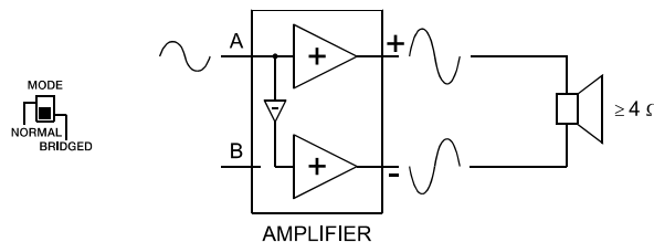
Abbildung 2.9: Betriebsart BRIDGED
