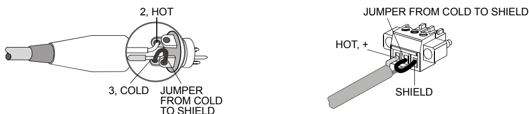
Illustration 2.11 : Connexion non-symétrisé de l'entrée
