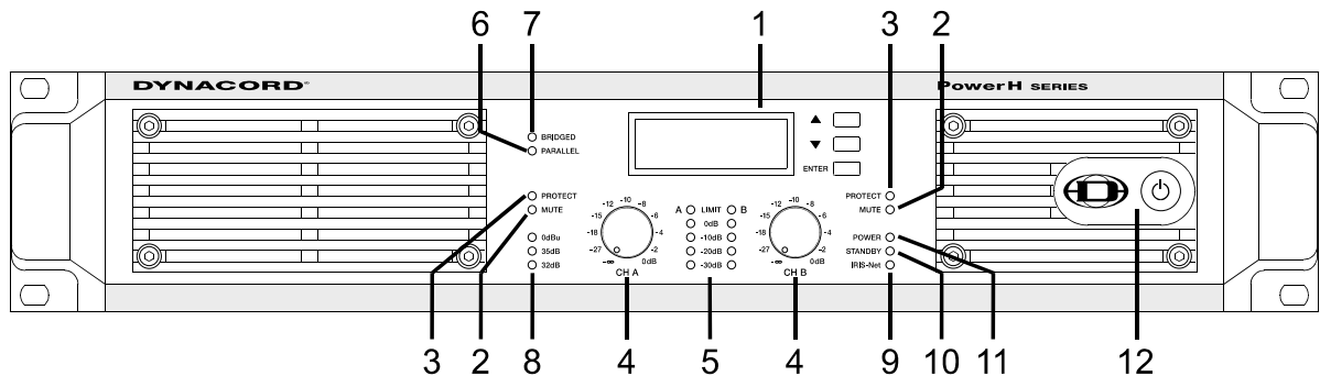
Abbildung 2.1: H2500/H5000 Frontseite
