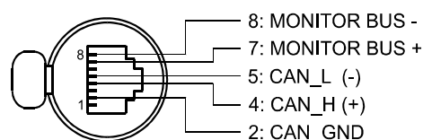
Abbildung 4.6: Belegung der CAN-Buchse
