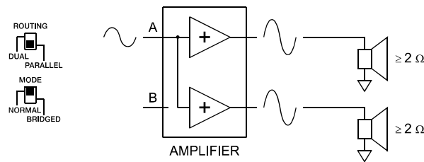
Illustration 2.8 : Signal audio appliqué au connecteur d'entrée A en mode PARALLEL
