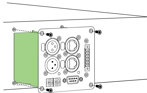
Abbildung 4.1: Einbau des RCM-26 in eine Endstufe
