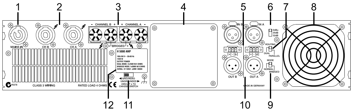
Illustration 2.2 : Arrière du H2500/H5000
