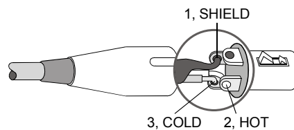
Abbildung 2.12: Symmetrische Beschaltung des Ausgang (Daisy-Chain)
