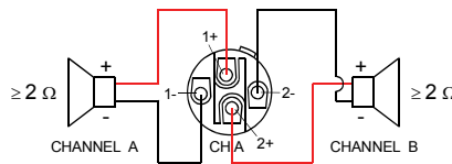
Abbildung 2.15: Bi-Amp-Lautsprecheranschluss in Betriebsart NORMAL nur an Speakon A
