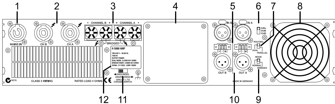
Abbildung 2.2: H2500/H5000 Rückseite
