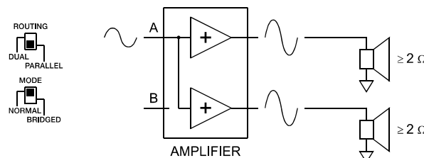
Abbildung 2.8: Einspeisung an Eingang A bei Betriebsart PARALLEL
