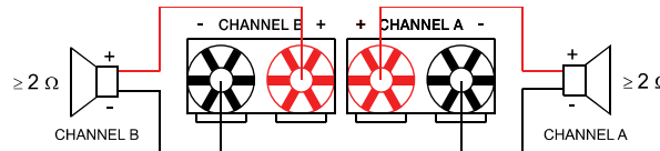
Illustration 2.14 : Connexion de haut-parleur en mode de fonctionnement NORMAL, à l'aide des bornes
