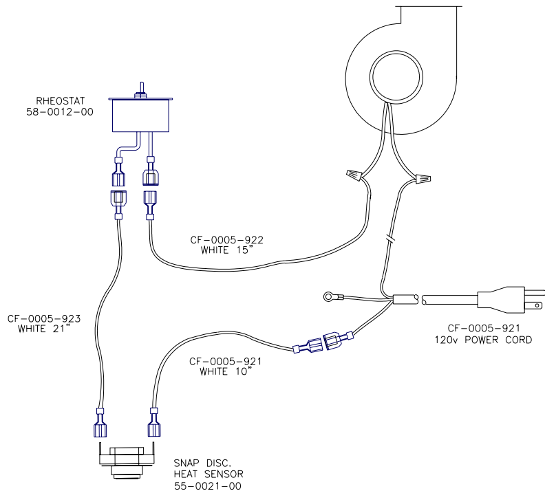
FIGURE 12: BLOWER FAN
