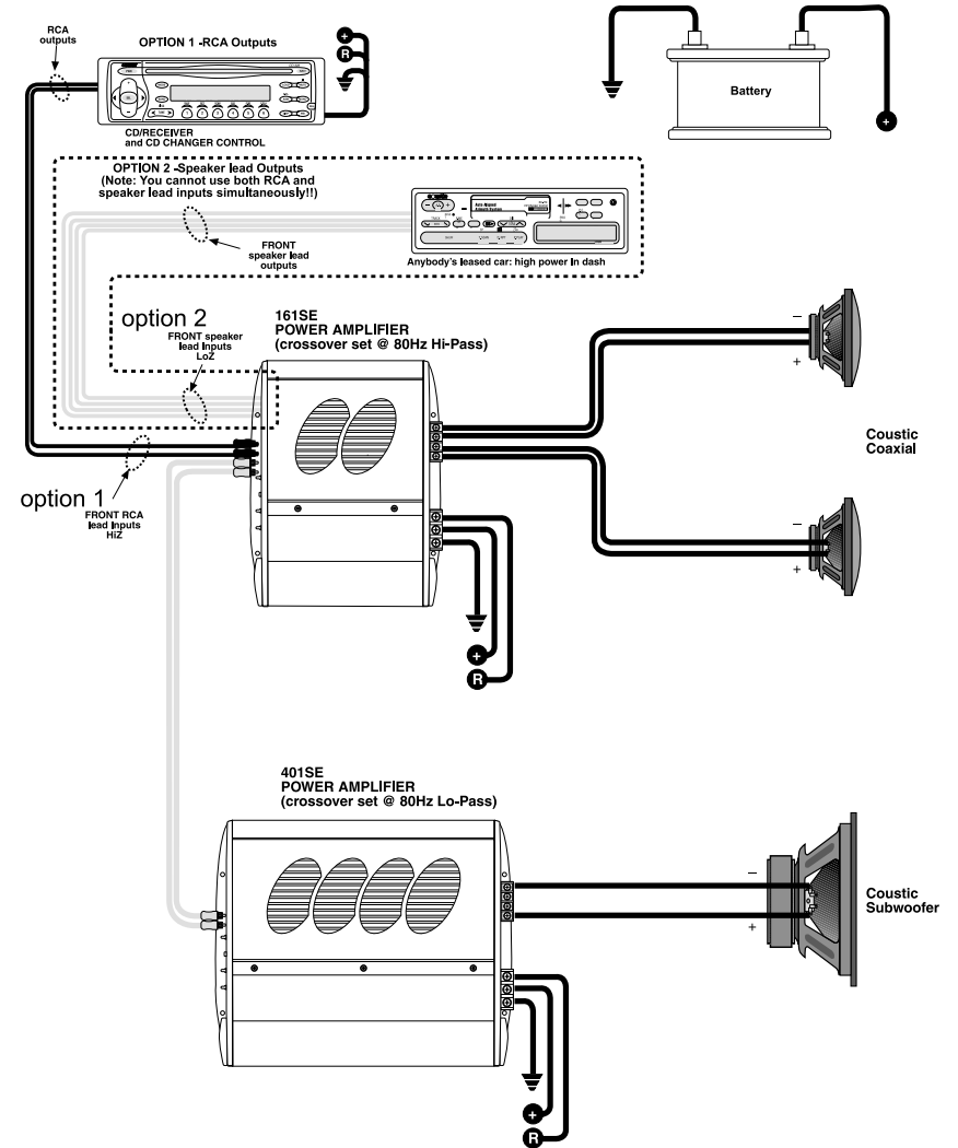
Figure 7 : Système multi amplifié
