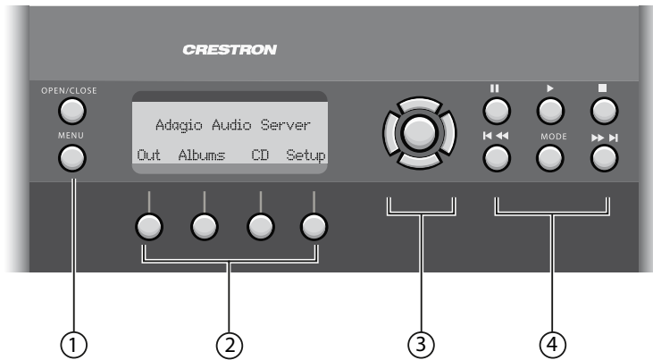
Abb. A - Anzeige auf der Vorderseite
