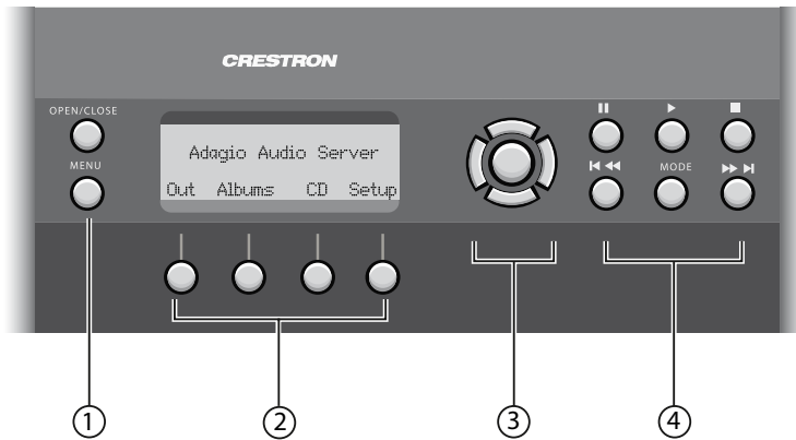
Fig. A - Ecran du panneau frontal
