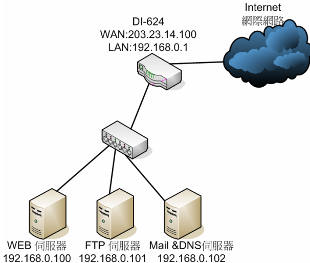
DI-624 虛擬伺服器設定範例,網路架構圖
