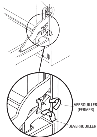
ROULEAU DE CHARNIÈRE DE PORTE
