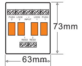
ILM-200 Interlock Module
