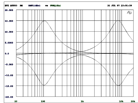
MID EQ
