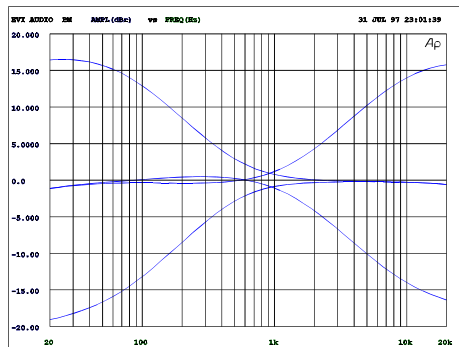
LO-HI EQ
