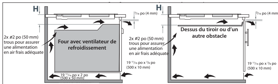
Fig. 1 Dégagements minimaux et exigences de ventilation - four installé sous la plaque de cuisson
