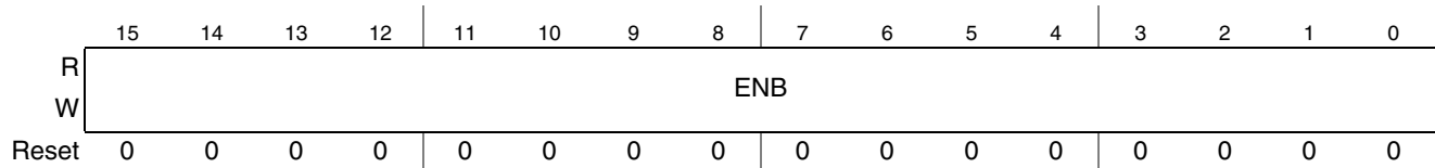
Figure 9-6. RGPIO Enable Register (RGPIO_ENB)
