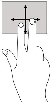
Figure 27. Défilement
