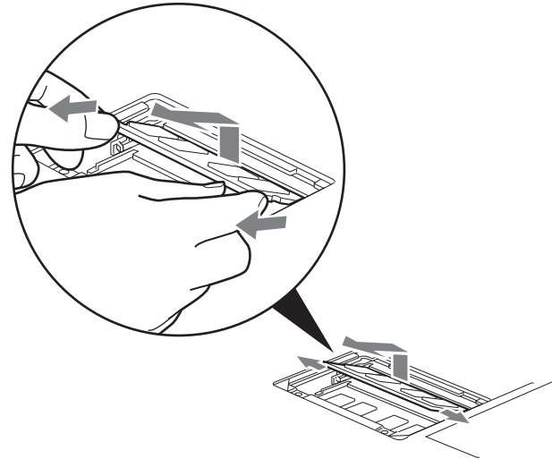
Figure 43. Retrait d'un module de mémoire
