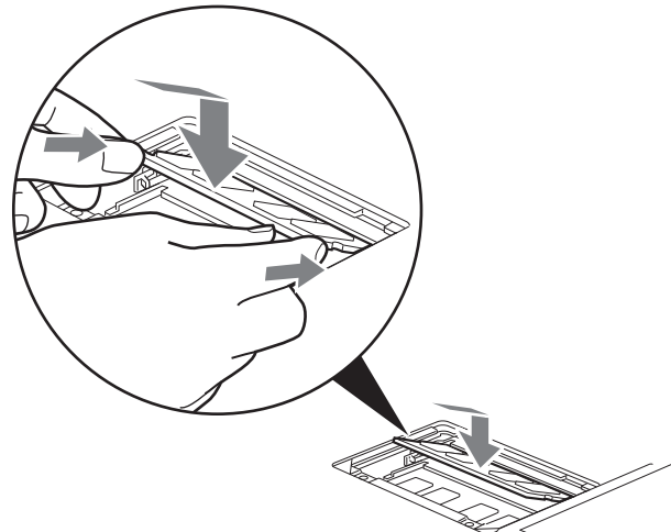
Figure 42. Installer un module de mémoire
