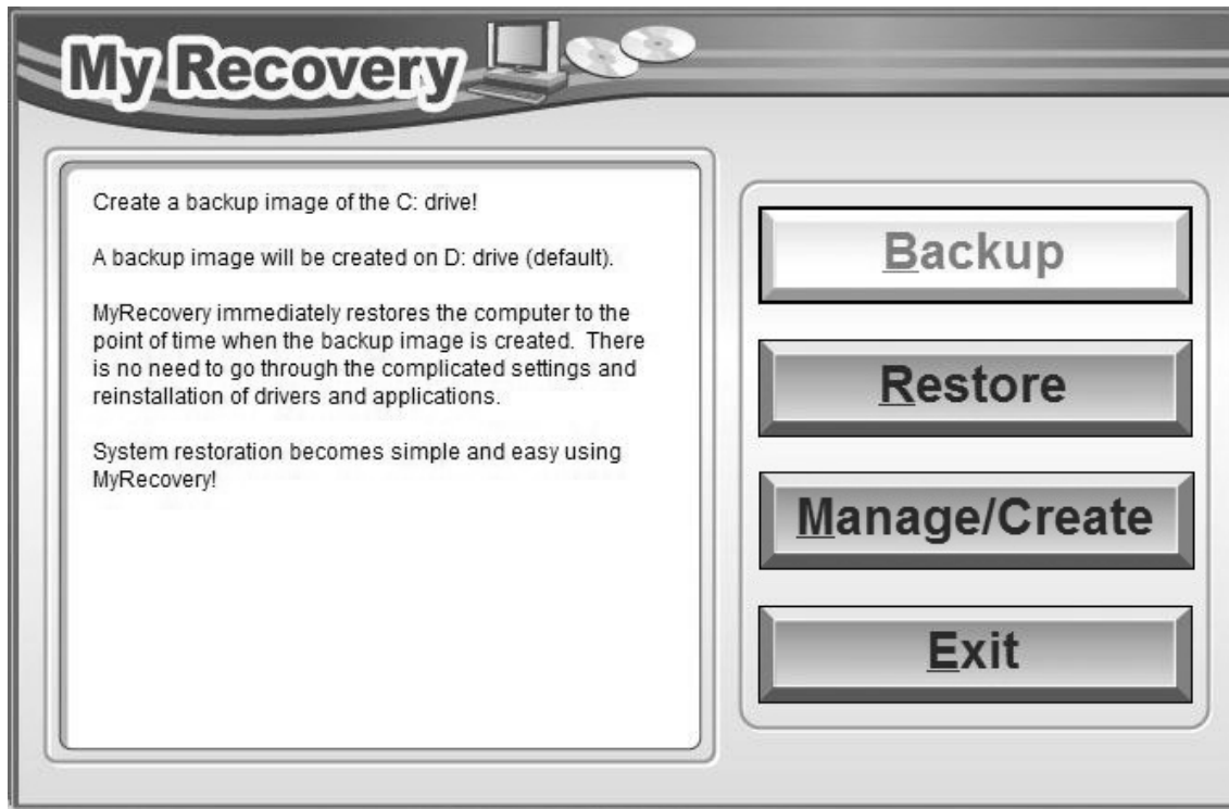
Figure 52. Écran MyRecovery
