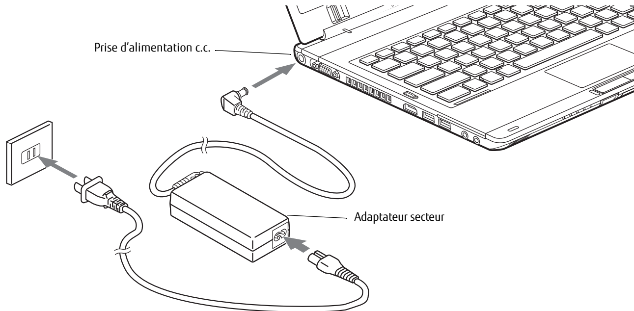
Figure 36. Connexion de l'adaptateur secteur
