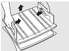
Cómo desarmar la bandeja de Enfriar / Descongelar
