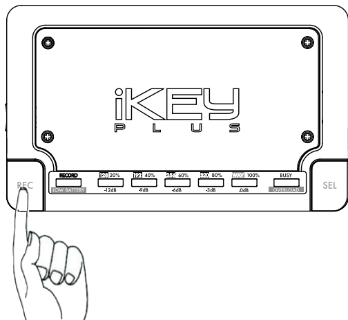
Figure E - Toutes les LEDs s'allumeront simultanément & rapidement 3 fois, indiquant que vous pouvez retirer le périphérique USB en toute sécurité.
