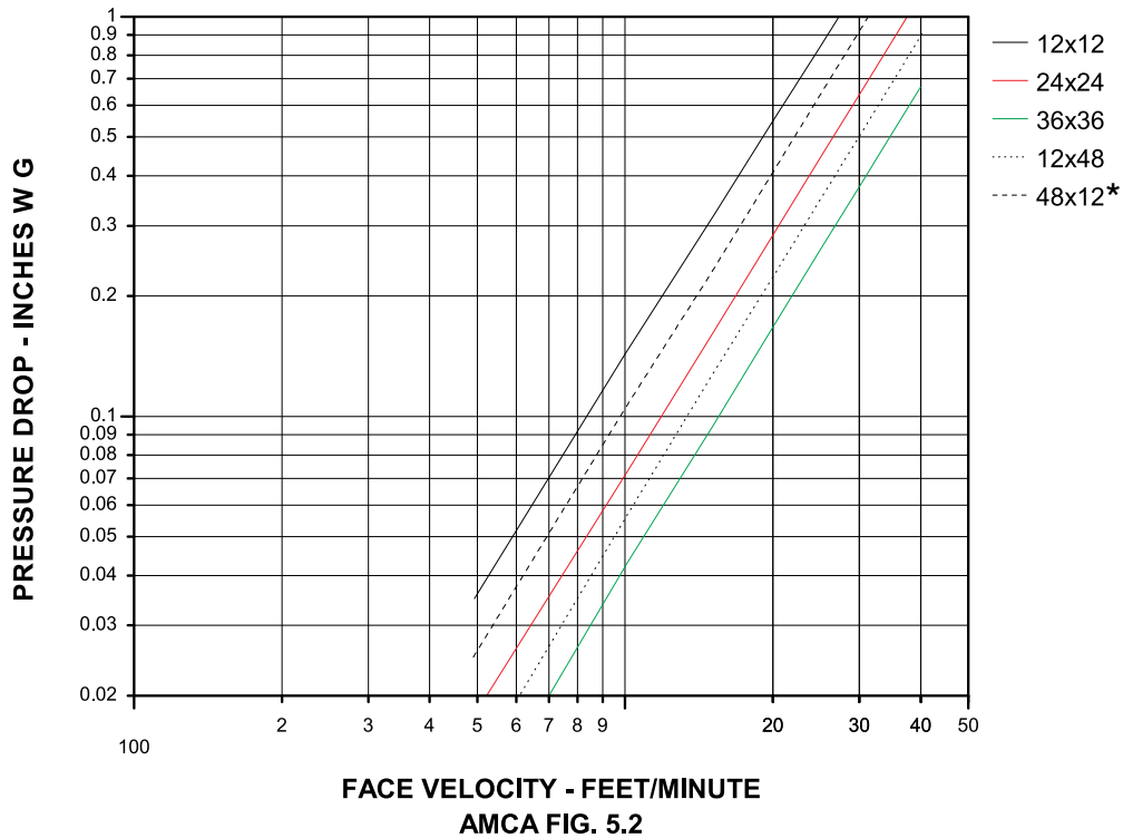
AMCA FIG. 5.2
