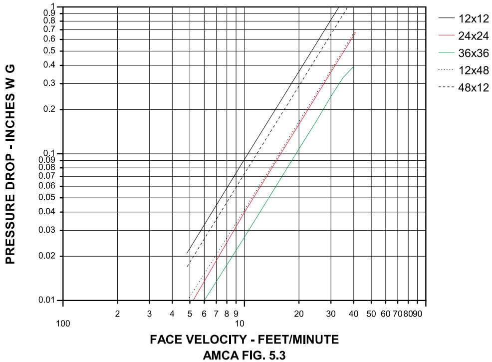
AMCA FIG. 5.3
