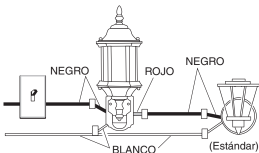
Conexión a la luz de movimiento y al aparato estándar
