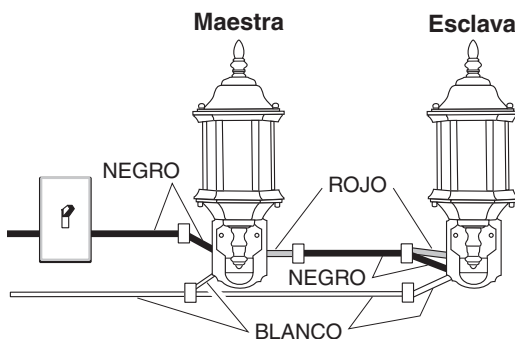
Conexión para controlar una luz de movimiento (esclava) desde otra (maestra)
