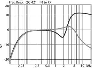
En la figura se muestran las curvas para PRESENCE (curva superior) y TREBLE (curva inferior) en los ajustes extremos del regulador HF-CHARACTER.
