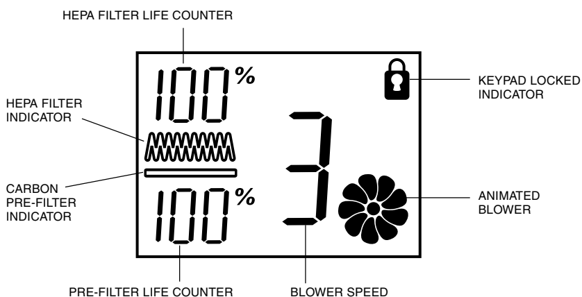
Fig. 5 - Alpha-numeric Display
