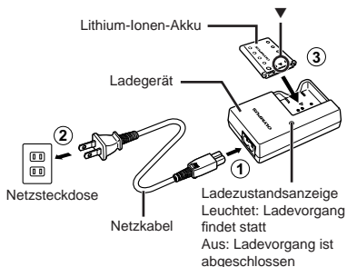
Ladegerät LI-41C
