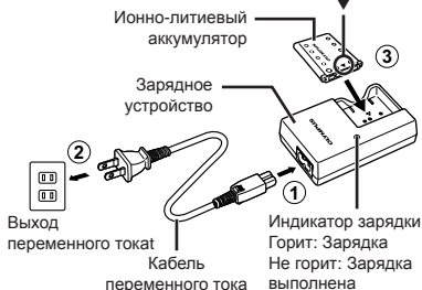
Зарядное устройство LI-41C
